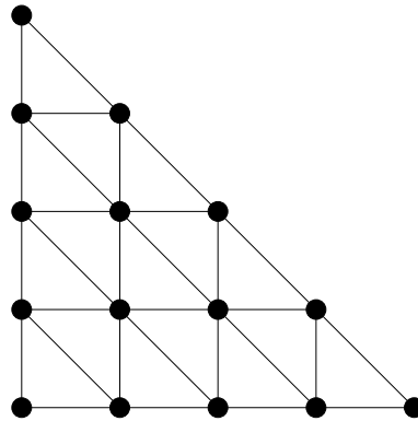
Abbildung 6.2.1: Triangulierung des Simplex in Subsimplices, die alle dem Ausgangssimplex ähnlich sind, aber nur ein Viertel der Größe haben. Ähnliche Unterteilungen gibt es in beliebigen Dimensionen, sie sind dann nur ein wenig komplizierter, siehe [3, 29].
