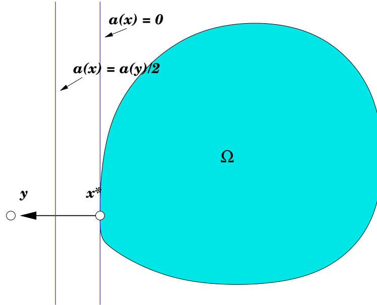
Abbildung 2.3.1: Konstruktion der Trennhyperebene: Zuerst findet man den Extrempunkt, dann liefert 2.3.11 bereits, daß die durch x^* gehende Gerade, die senkrecht auf y - x^* steht, eine schwache Trennfunktion hat: Mindestens ein Punkt von \Omega , nämlich x^* liegt noch auf dieser Hyperebene – aber der Punkt ist auch eindeutig, wenn die Menge \Omega strikt konvex ist. Schieben wir sie nun ein bißchen in Richtung y – der Wert \frac{1}{2} war hier total willkürlich – dann sind beide Ungleichungen der Trennung so strikt wie in 2.3.9 gefordert.
