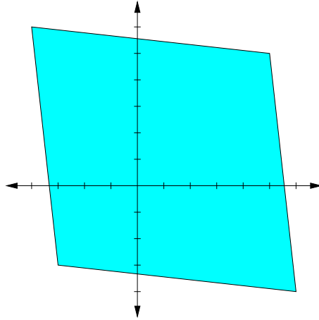
Abbildung 5.5.1: Der Auszahlungsbereich \Gamma(A) = \Omega(A) zum „offiziellen“ Gefangenendilemma.
