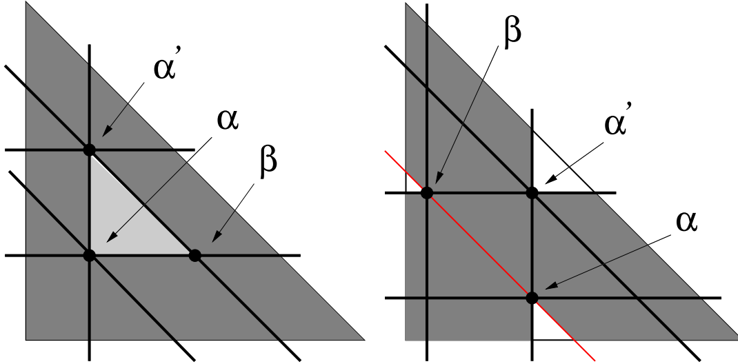
Abbildung 7.5.4: (Links) Der Punkt \beta aus 7.5.3 ist keine hilfreiche Erweiterung von \alpha und \alpha' , da der hellgraue Bereich immer noch undominiert bleibt. (Rechts) Die Auswahl \beta stimmt schon optimistischer, allerdings bleiben immer noch drei kleine Dreiecke weiß, aber das kann man ja beheben, indem man \alpha ganz nach unten, \alpha' ganz nach oben und \beta ganz nach links schiebt.
