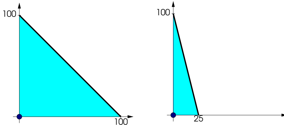
Abbildung 5.2.2: Die Bereiche \Omega(A) zu Beispiel 5.2.5 ( links ) und dessen Variante (5.2.4). Der Auszahlungsbereich besteht nur aus der fetten Linie und dem Nullpunkt, erst durch die konvexe Hülle und die damit verbundenen gemeinsamen Strategien gewinnt er wirklich an Dimension.
